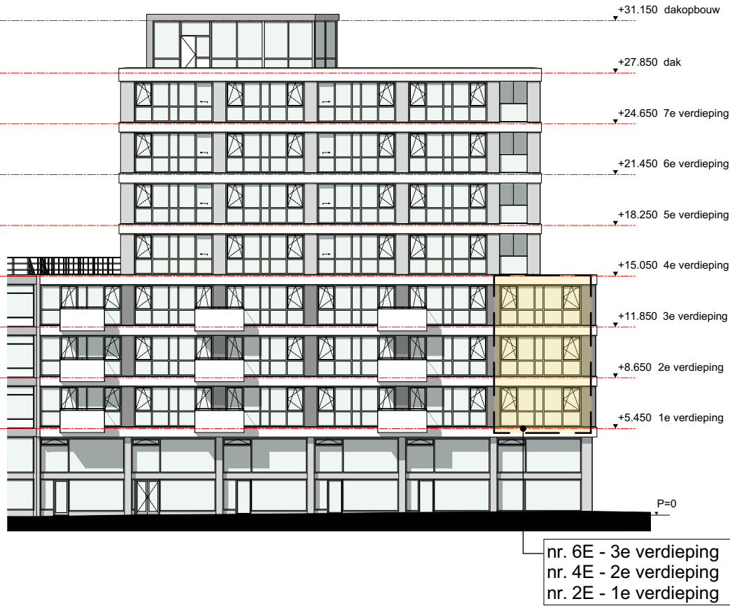
gevel Hoogstraat
